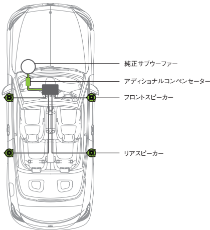
SC-A205M 4スピーカーモジュール システム構成図
