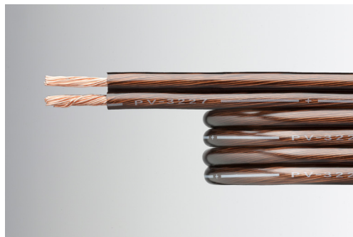
スピーカーケーブル「PV-3227」（切断面イメージ写真）
